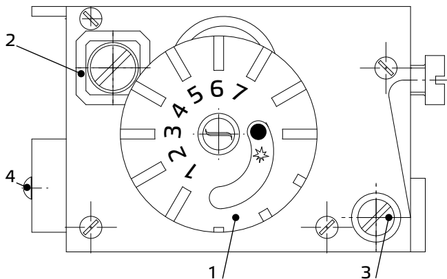
Рисунок 2 — Блок газовый
