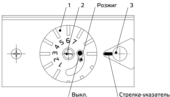
Рисунок 2 — Блок газовый
